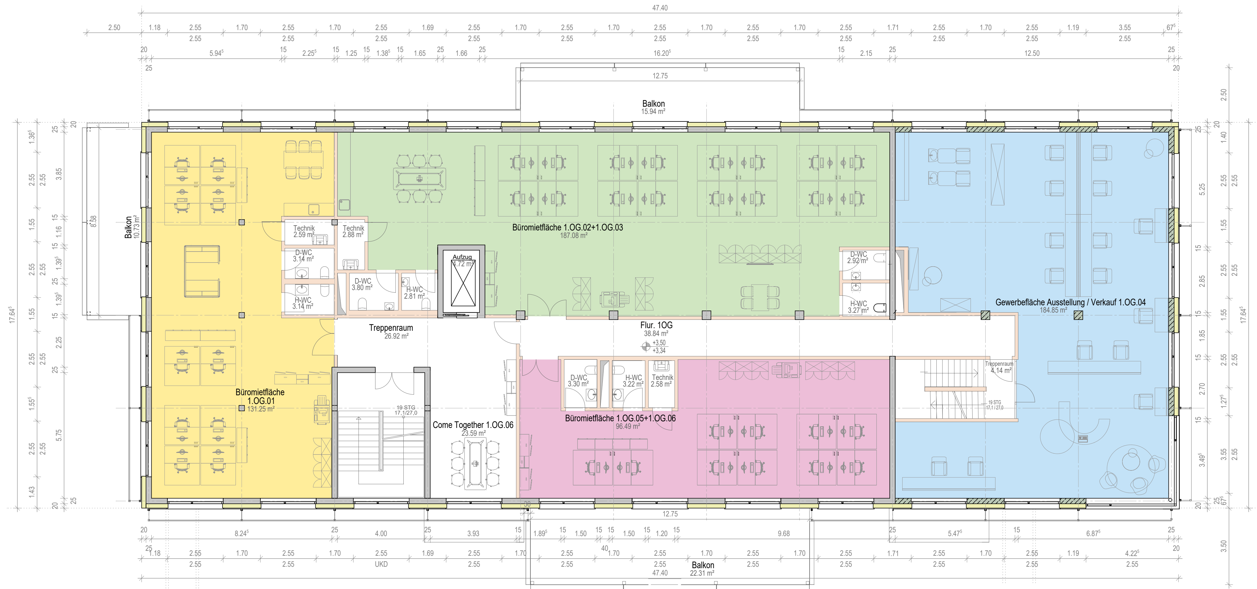
Grundriss 1. Obergeschoß - 1. Bauabschnitt M 1:100
